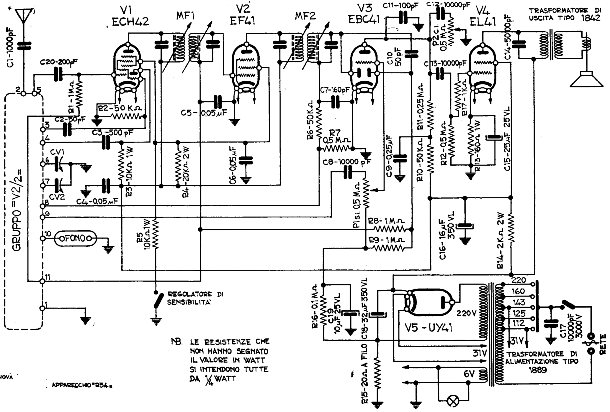
NOVA - Mod. R54. Ricevitore con sintonia a permeabilità variabile provvisto di gruppo AF mod. V 2/2. Media frequenza 465 kc/s. Potenza indistorta di uscita 3,5 watt. Consumo 40 watt.
